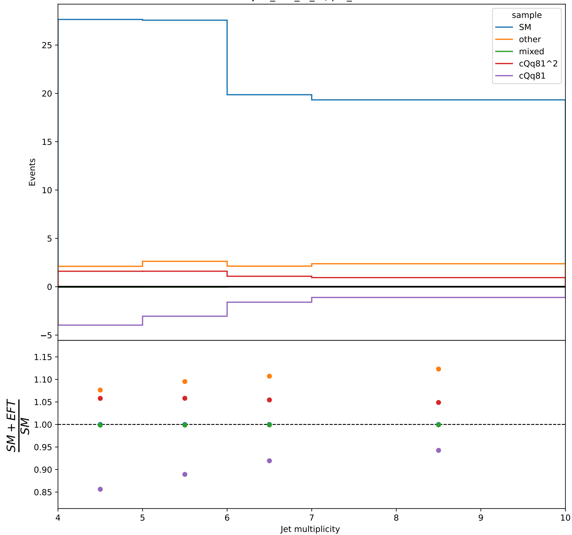
njets_2lss_4t_cQq81_-0.85
