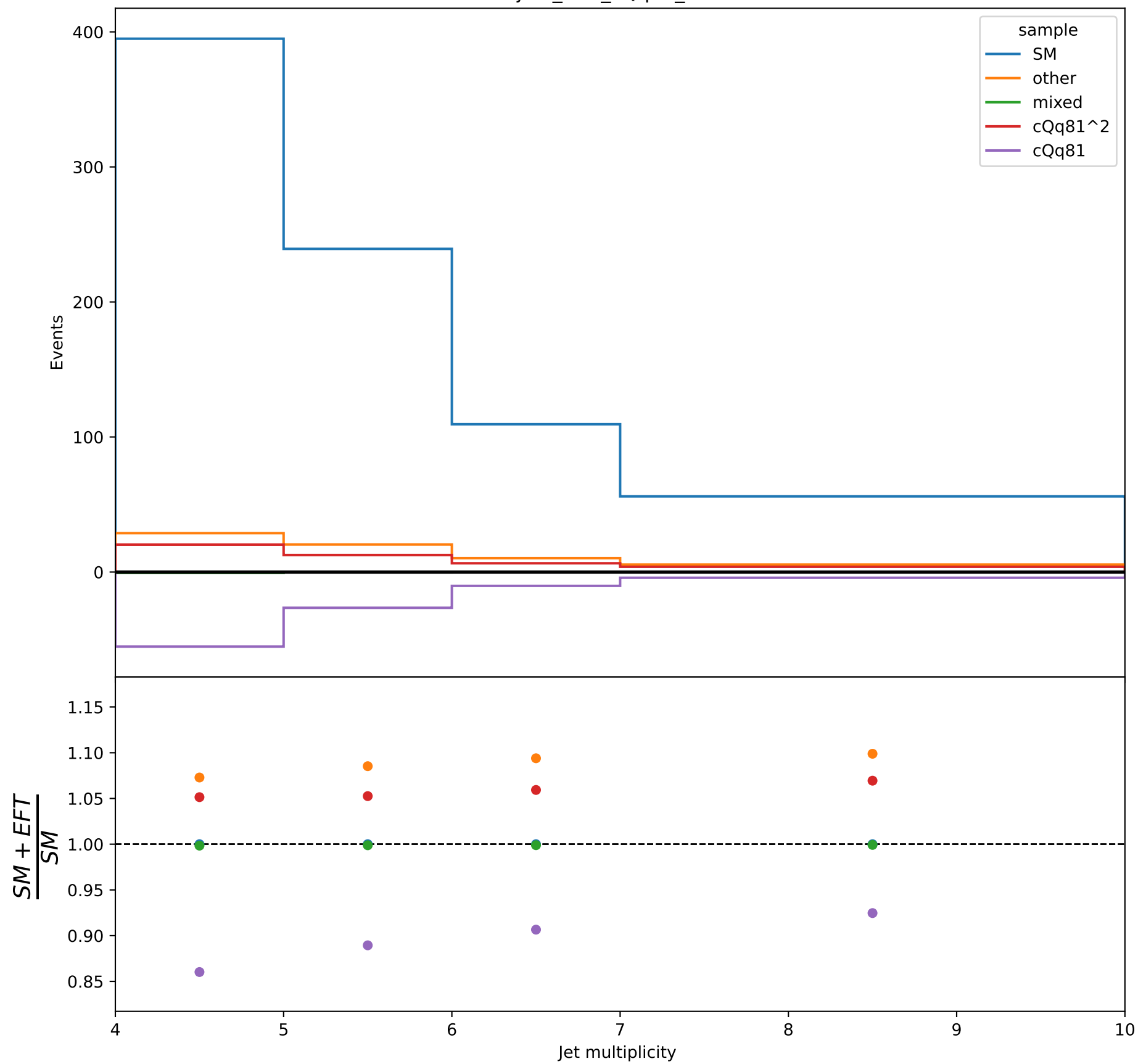
njets_2lss_cQq81_-0.85
