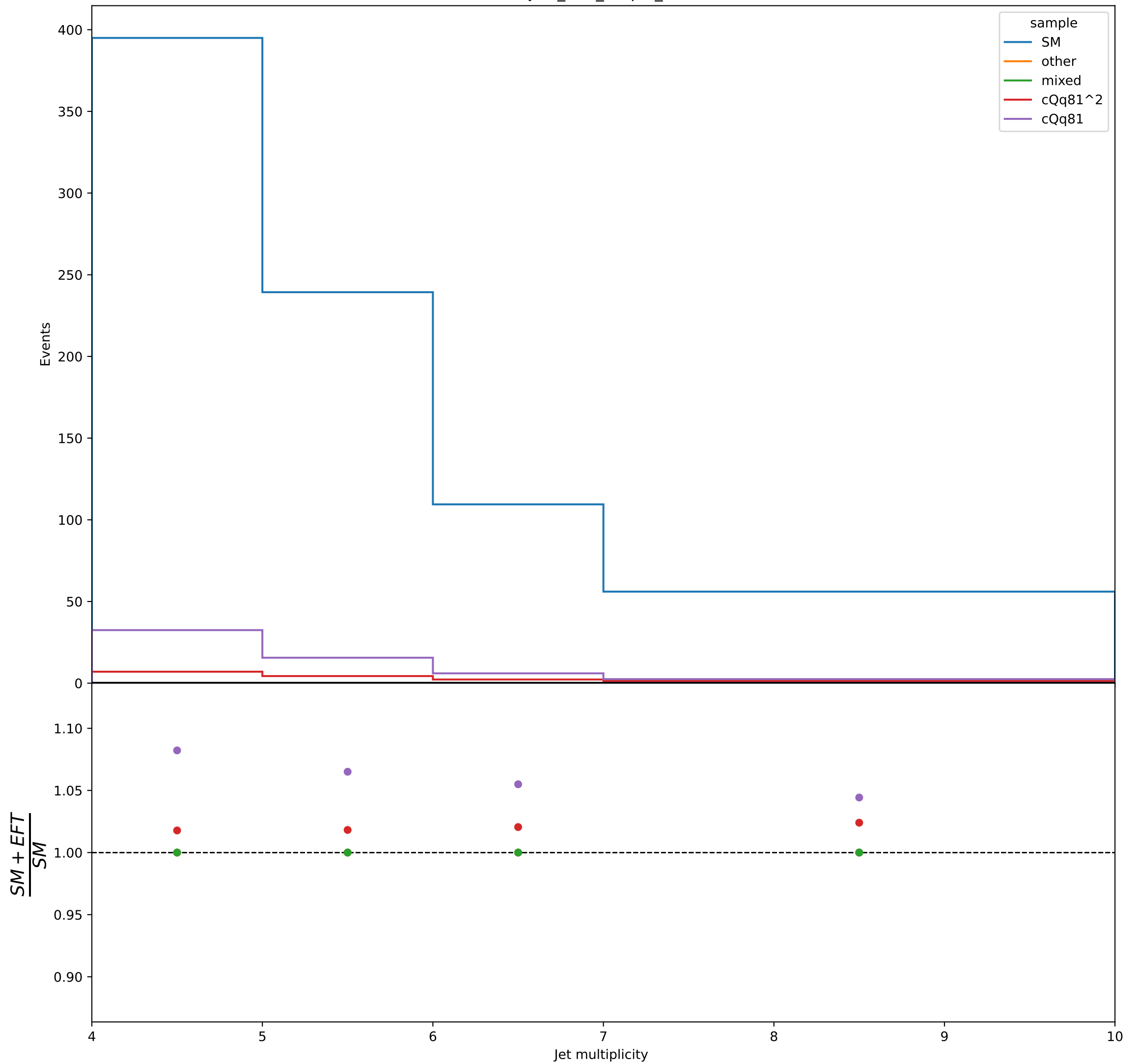
njets_2lss_cQq81_0.5
