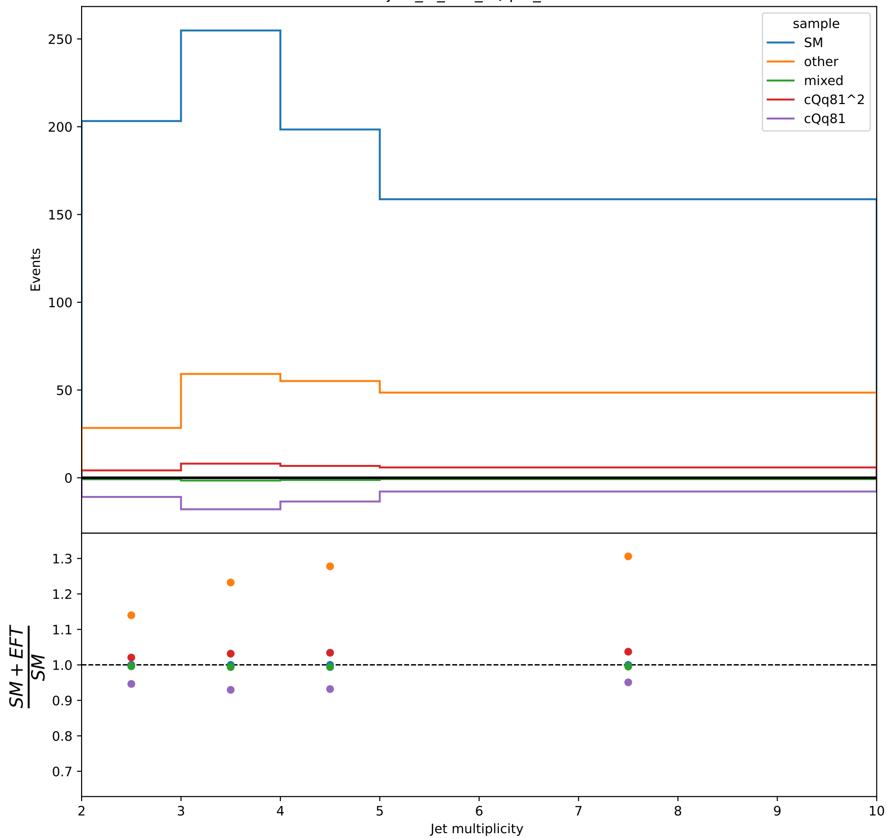
njets_3l_onZ_cQq81_-0.85
